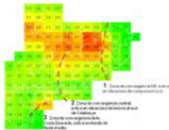
Figura 8: Actividad eléctrica según AEMET-Sinobas (a) (Densidad anual de descargas eléctricas (Número de descargas / km 2 ) 2003-2012 ) y Meteocat (b) Densidad de rayos (rayos NT km -2 año -1 ) En una cuadrícula de 20 x 20 km, media del período 2004-2008.
